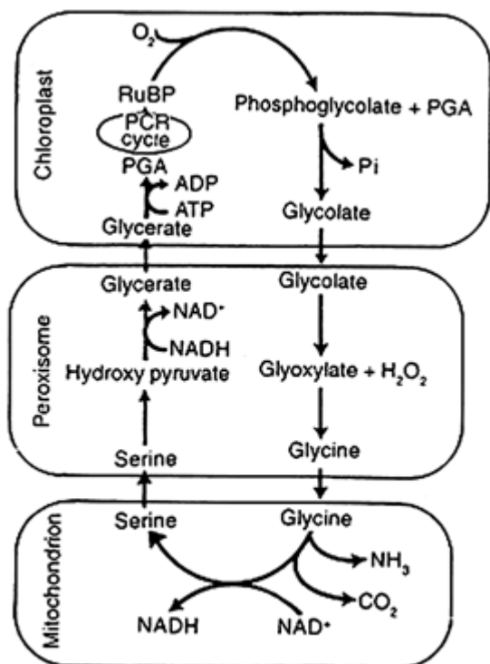
Fig. 5.10. Photorespiration.
